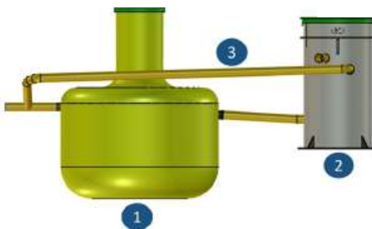
1 - Usazovací nádrž 2 - Čistírna OV 3 - Potrubí pro návrat kalu
